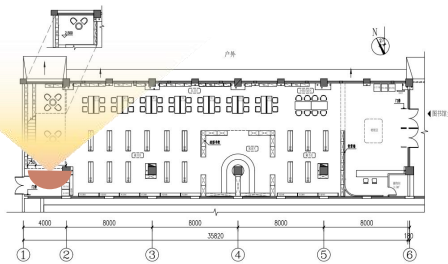
图书馆方案平面图
